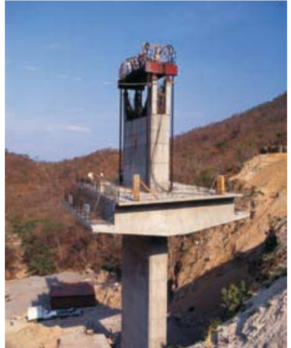
Puente El Pozuelo, Carr. México-Acapulco
