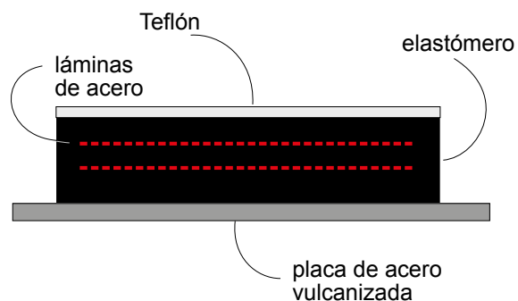
Apoyo Elastomérico deslizante
